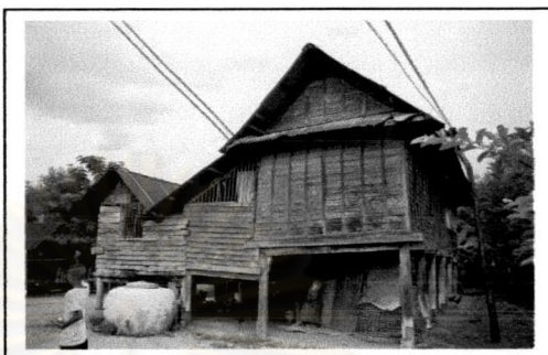
ภาพที่ 5.15-16 แสดงการแบ่งระดับและการใช้พื้นที่ได้ถุน ของเรือนไท-โคราช ที่มา ภาพโดยนายธีรชัย ลีสุระพลานนท์ ธันวาคม 2546
