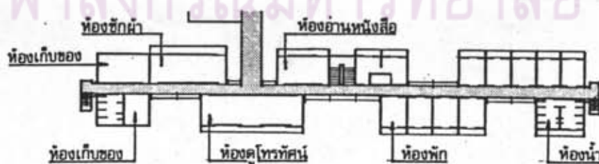
ผังชั้นล่างอาคารหอพักวิทยาเขตศาลายา
