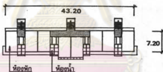
ผังชั้นบนอาคารหอพักแบบที่ ๑ วิทยาเขตกำแพงแสน
