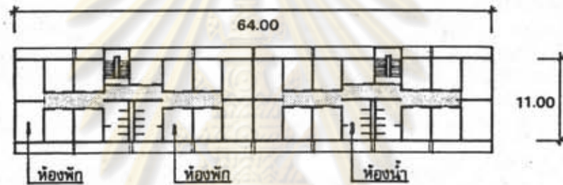
ผังชั้นบนอาคารหอพัก A1 วิทยาเขตทับแก้ว
