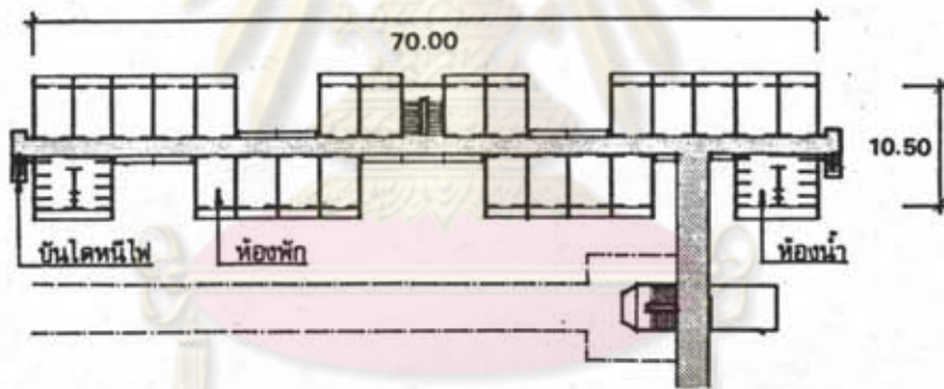
ผังชั้นบนอาคารหอพักวิทยาเขตศาลายา
