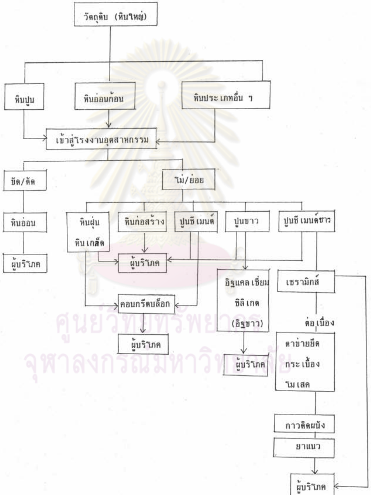
แผนภูมิที่ 8 แสดงขบวนการผลิตวัสดุก่อสร้างในจังหวัดสระบุรี
