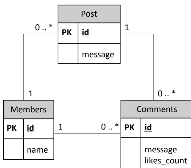
ภาพที่ 4.1 แผนภาพอีอาร์ (ER Diagram)
