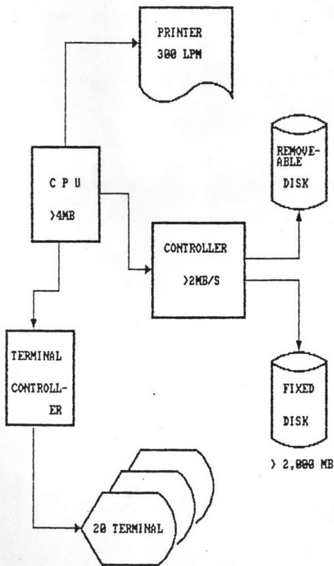
- แผนภาพที่ 4.2 แสดงอุปกรณ์ของเครื่องคอมพิวเตอร์ขนาดกลางสำหรับระบบงานใหม่
