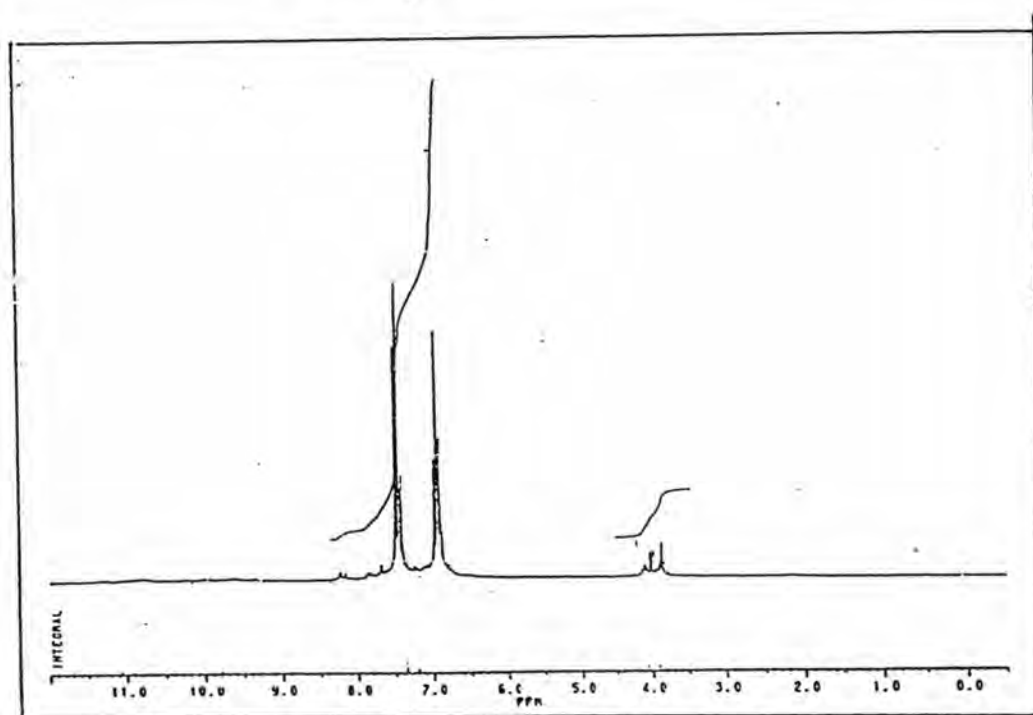
Fig. 52a: IR spectrum of Dye 8
