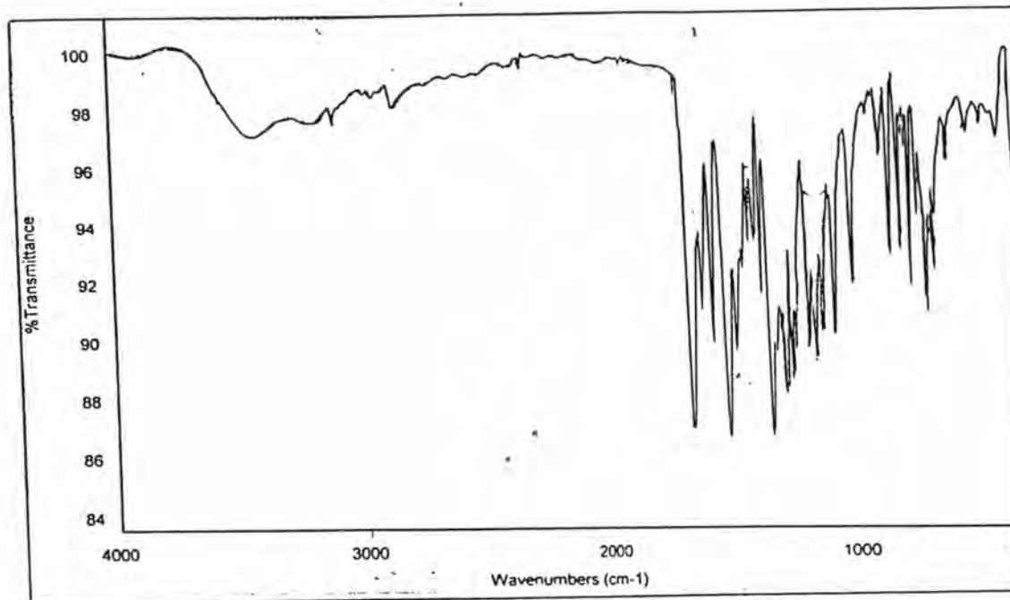
Fig. 52a: IR spectrum of Dye 8
