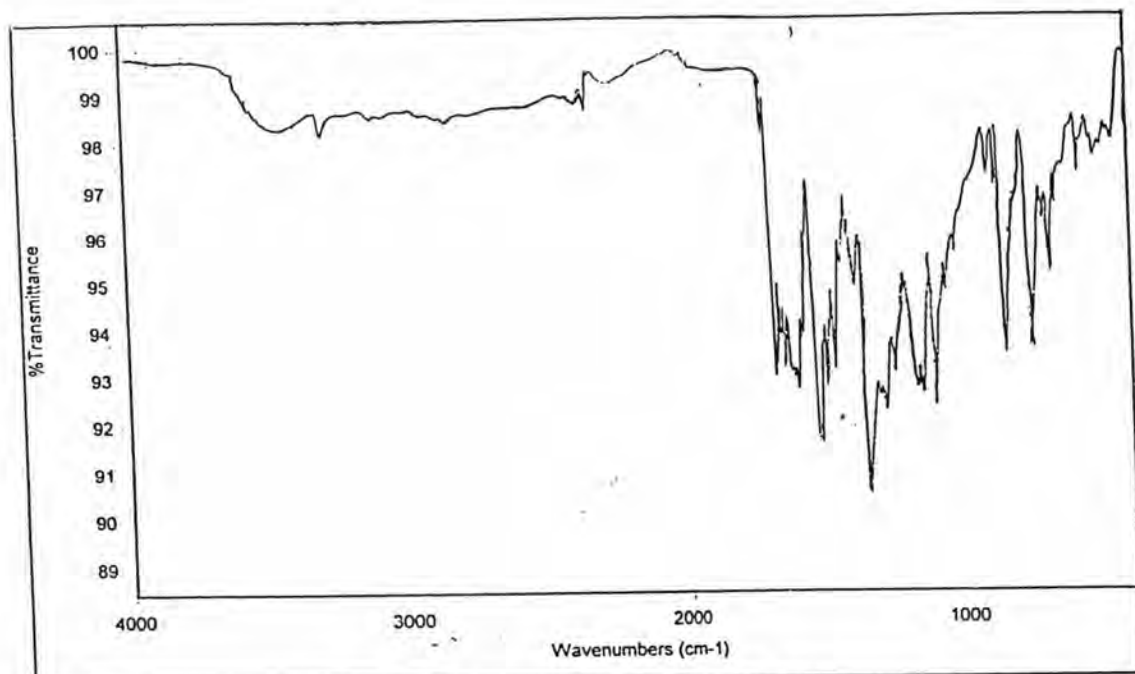
Fig. 58a: IR spectrum of Dye 2
