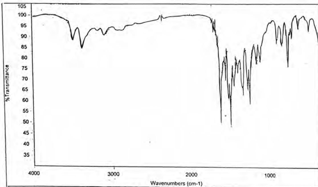
Fig. 46a: IR spectrum of Dye 7
