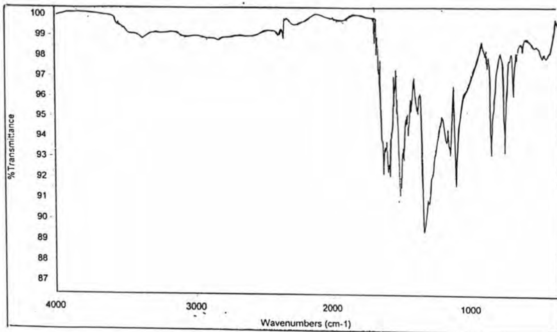
Fig. 34a: IR spectrum of Dye 5
