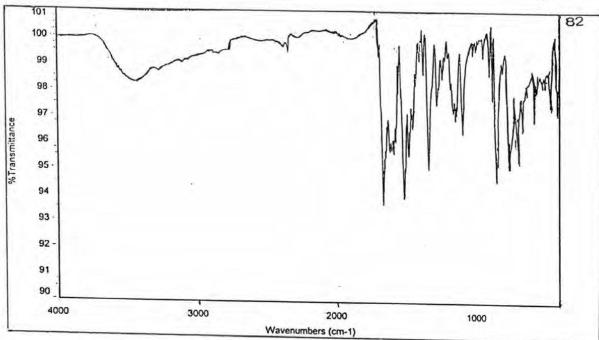
Fig. 10a: IR spectrum of Dye 1
