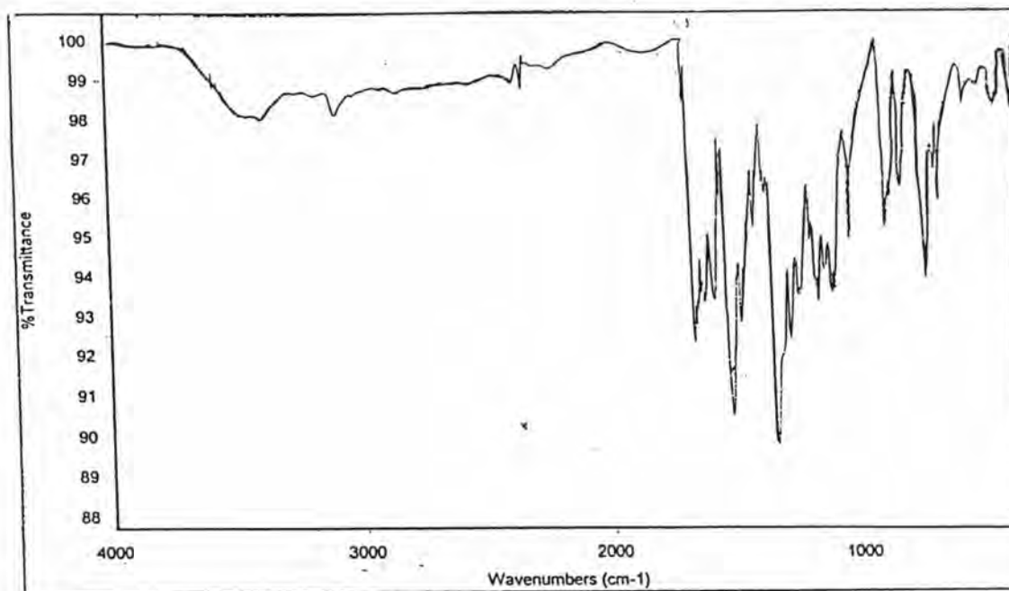
Fig. 40a: IR spectrum of Dye 6
