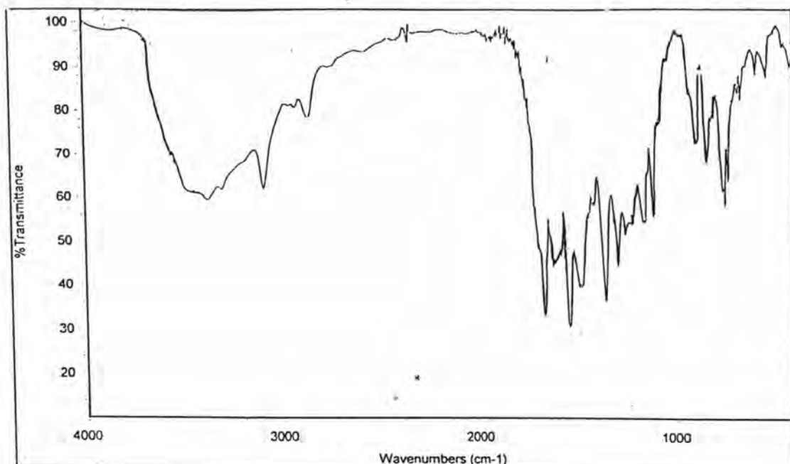
Fig. 22a: IR spectrum of Dye 3
