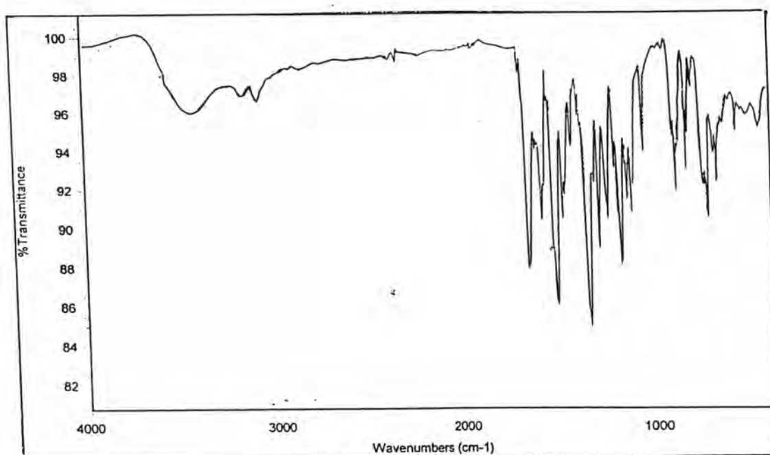
Fig. 28a: IR spectrum of Dye 4
