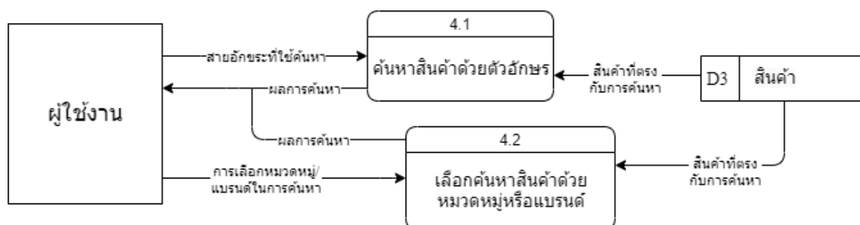
ภาพที่ 3.7 แผนภาพการไหลของข้อมูล ระดับ 1 : ค้นหาสินค้า
