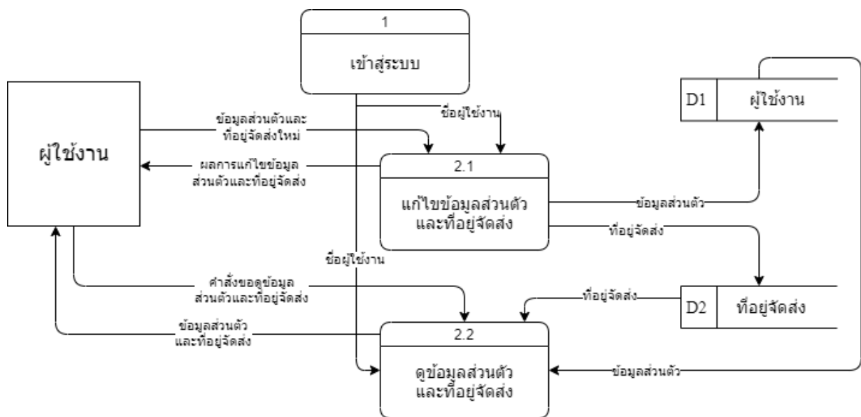
ภาพที่ 3.6 แผนภาพการไหลของข้อมูล ระดับ 1 : จัดการข้อมูลส่วนตัวและที่อยู่จัดส่ง
