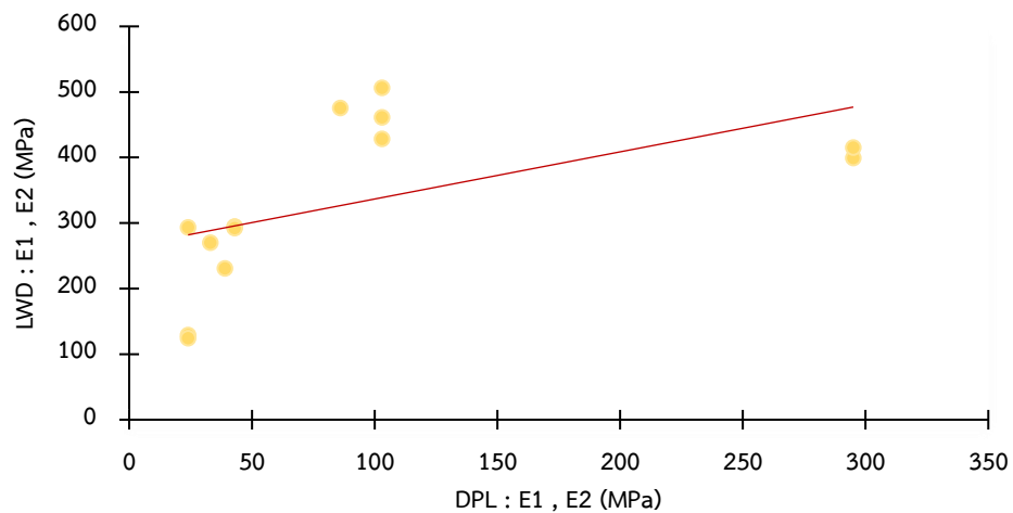
รูปที่ 70 การเปรียบเทียบค่าโมดูลัสยืดหยุ่นของชั้นทางจากผลการทดสอบด้วย เครื่องมือ LWD และ DPL
