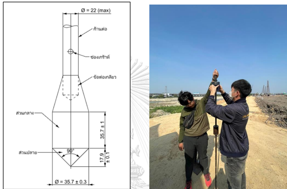
รูปที่ 26 เครื่องมือ Dynamic Probing Light
