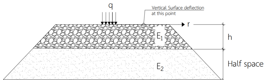
รูปที่ 15 ระบบสองชั้นทาง (Huang, 1969)
