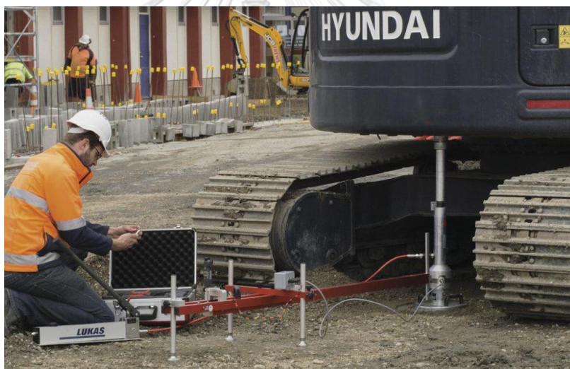
รูปที่ 2 การทดสอบ Plate load test (New Zealand Geotechnical Society)
