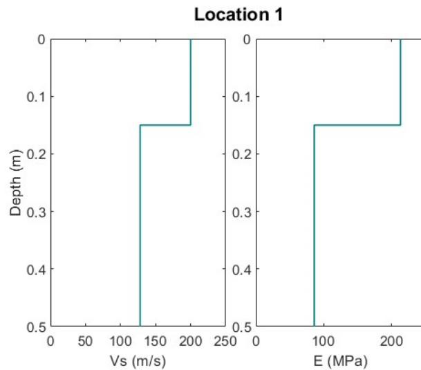
รูปที่ 57 หน้าตัดความเร็วคลื่นเฉือน (Vs Profile) แปลงทดสอบที่ 1
