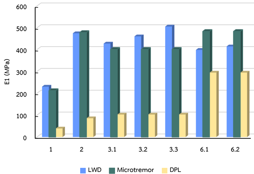
รูปที่ 71 แผนภูมิแท่งเปรียบเทียบค่าโมดูลัสยืดหยุ่นชั้นแรก ( E_1 ) ของวัสดุโครงสร้างทางแบบไม่เชื่อมแน่น
