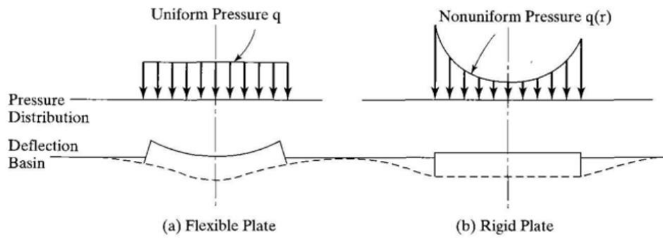
รูปที่ 16 ความแตกต่างระหว่างแผ่นงานโลหะแบบยืดหยุ่นและแบบแข็ง (Huang, 1969)
