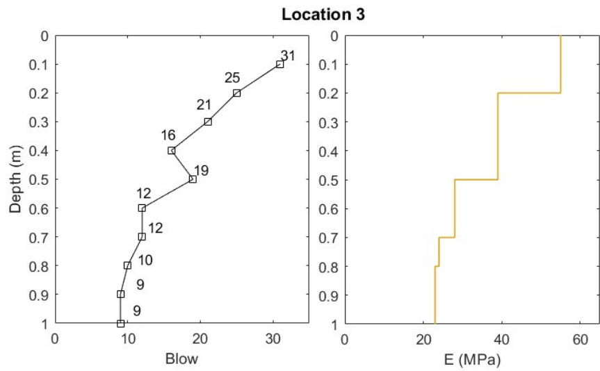
รูปที่ 55 ผลการทดสอบจากเครื่องมือ DPL ของแปลงทดสอบที่ 3
