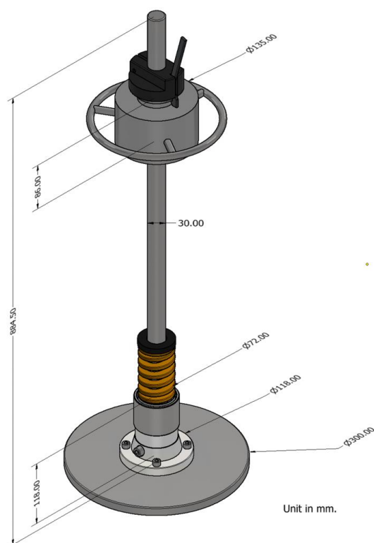
รูปที่ 20 เครื่องมือ LWD แบบมาตรฐาน
