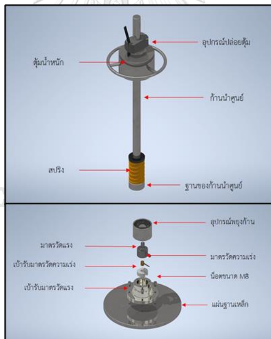
รูปที่ 25 รายละเอียดเครื่องมือ LWD
