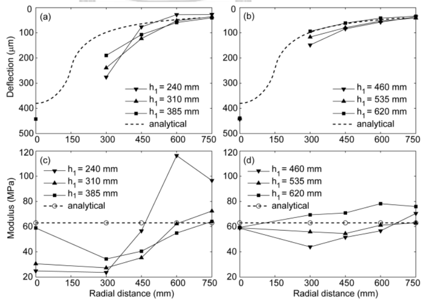
รูปที่ 23 แองการแอ่นตัวและโมดูลัสยืดหยุ่นที่ระยะต่างๆของ TB2-1 สำหรับตุ้มน้ำหนัก 10 kg
