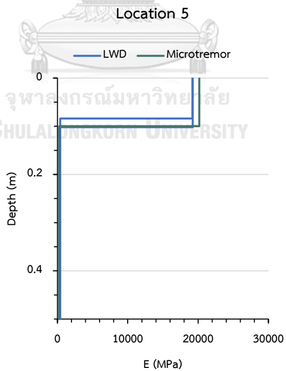
รูปที่ 67 ความสัมพันธ์ระหว่างค่าโมดูลัสยืดหยุ่นและความลึกของแปลงทดสอบที่ 5
