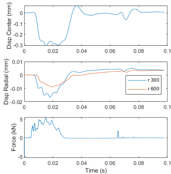
รูปที่ 52 ผลการตอบสนองที่ได้จากเครื่องมือ LWD ที่มีจีไอโฟนเพิ่มเติมในแนวนอน
