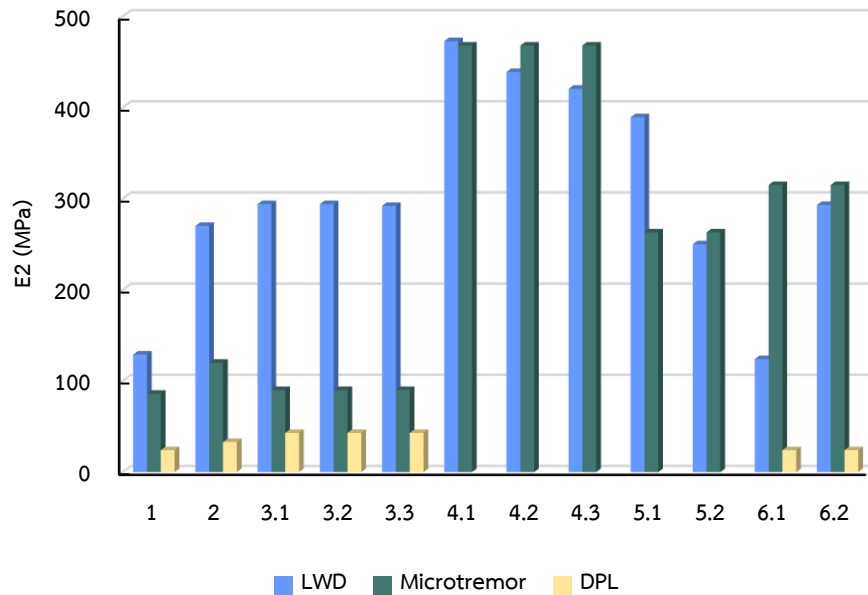
รูปที่ 72 แผนภูมิแท่งเปรียบเทียบค่าโมดูลัสยืดหยุ่นชั้นสอง ( E_2 ) ของวัสดุโครงสร้างทางแบบไม่เชื่อมแน่น
