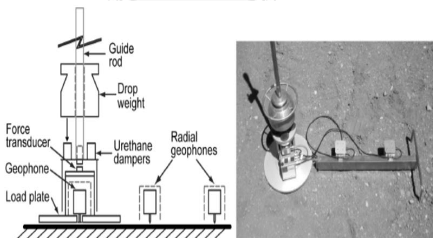
รูปที่ 10 เครื่องมือ Light Weight Deflectometer ติดตั้งเซนเซอร์วัดความเร็วคลื่นจำนวน 2 ตัว (Senseny & Mooney, 2010)
