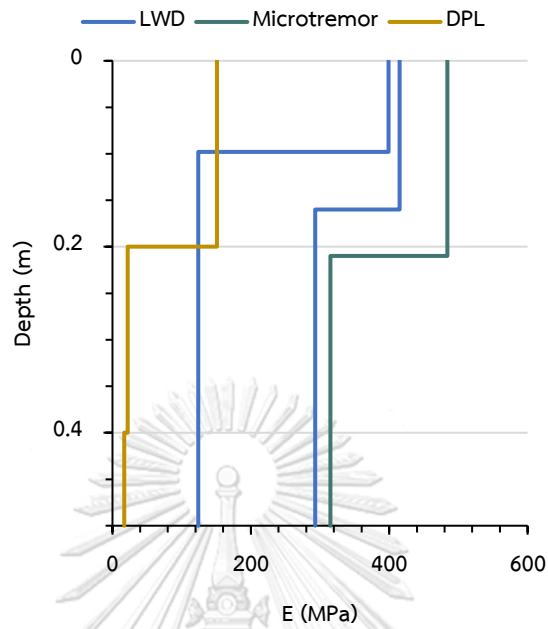
รูปที่ 68 ความสัมพันธ์ระหว่างค่าโมดูลัสยืดหยุ่นและความลึกของแปลงทดสอบที่ 6
