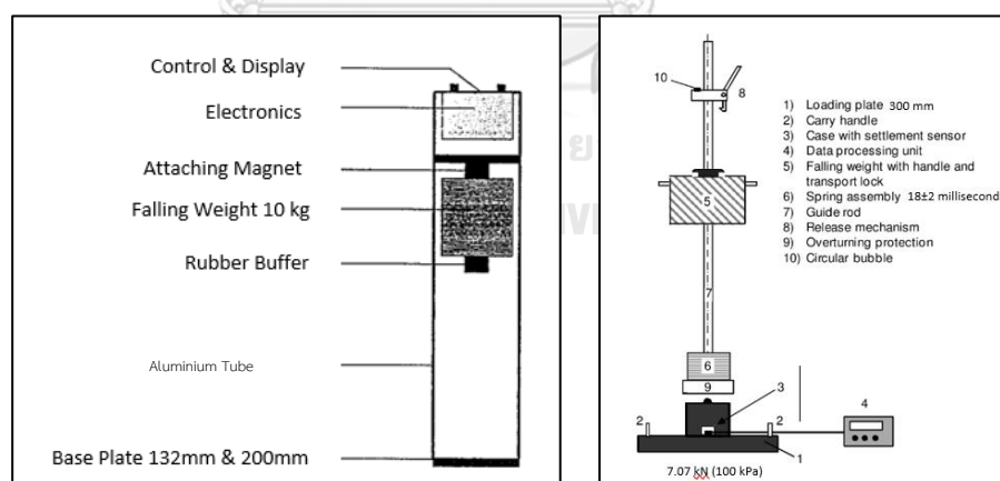
a) Loadman (Livneh, 1997)
