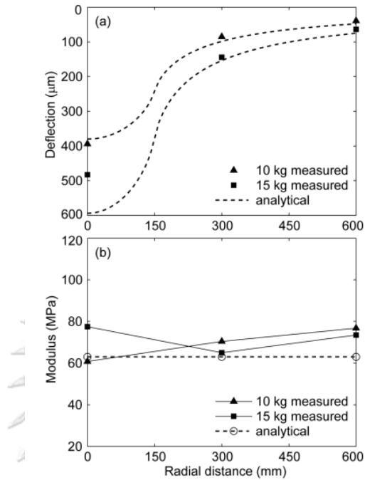
รูปที่ 22 (a) แองการแอ่นตัวที่ระยะต่างๆของ TB1-1 (b) ค่าโมดูลัสยืดหยุ่นที่ระยะต่างๆของ TB1-1
