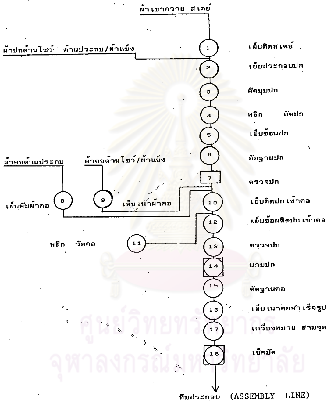
รูปที่ 3.6 กรรมวิธีในการเย็บผ้าของหน่วยปก (Collar Section)
