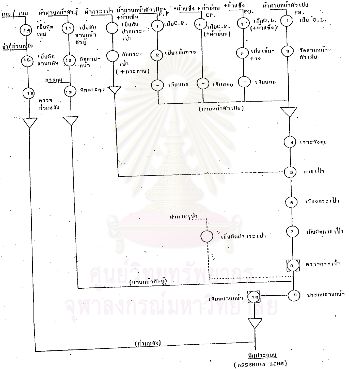
รูปที่ ๑.๑ การวิเคราะห์การเดินสายของหน่วยลำตัว (Body Section)
