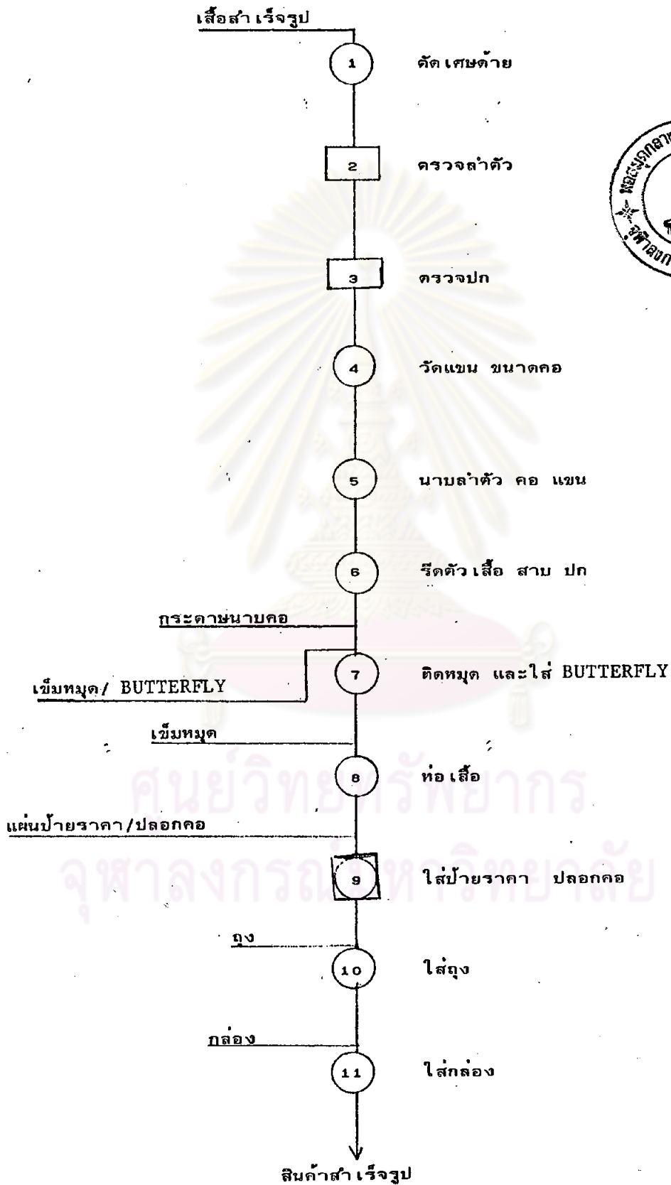
รูปที่ 3.11 กรรมวิธีการตกแต่งของหน่วยตกแต่ง (Finishing Section)
