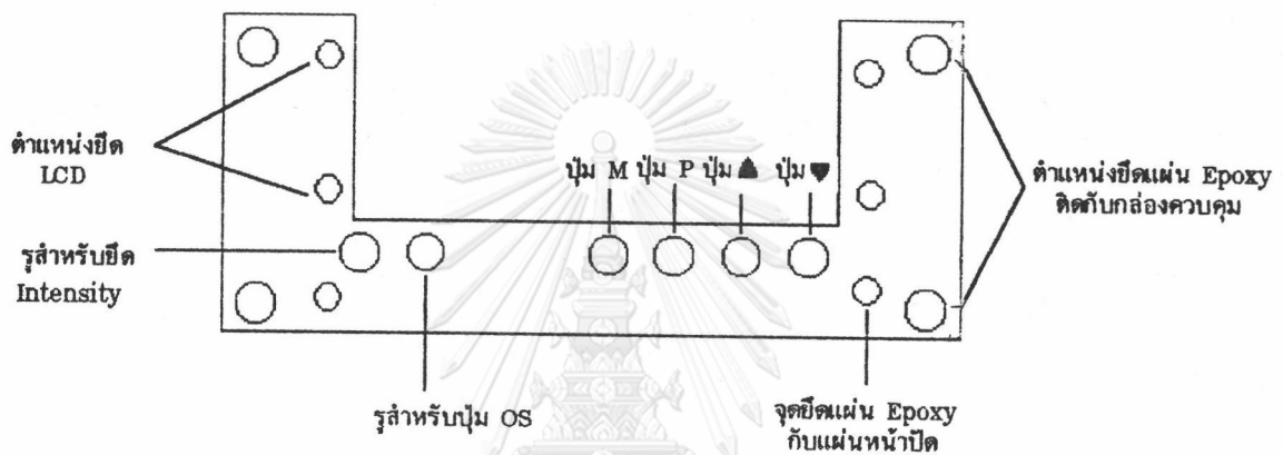
รูปที่ 5.4 แสดงรูปแบบของแผ่น Epoxy ที่ใช้เป็นโครงสร้างรองรับแผงหน้าปิด
