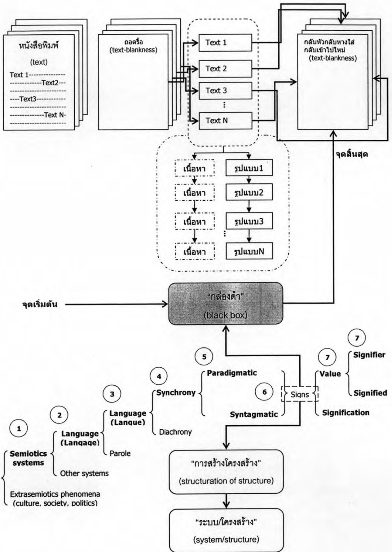
รูปที่ 24 แสดงกระบวนการศึกษาหนังสือพิมพ์ด้วยวิธีการแบบโครงสร้างนิยมและสัญวิทยา
