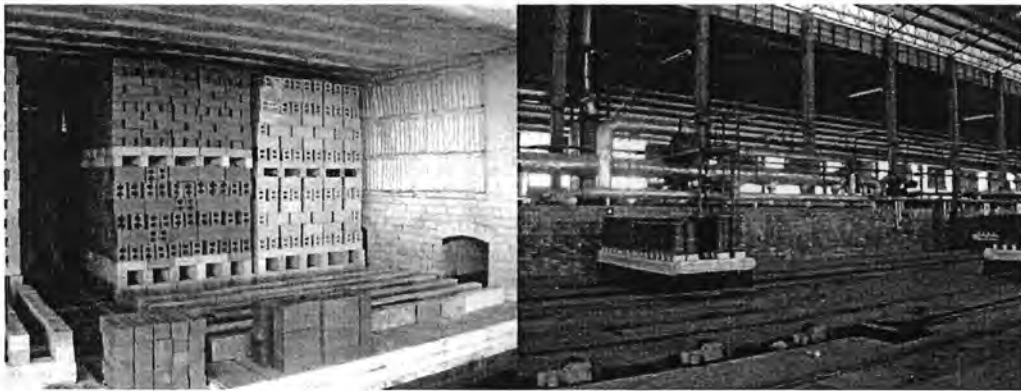
รูปที่ 3.87 เตาแก๊ส LPG มีลักษณะเป็นเตาอุโมงค์ที่ใช้งานอยู่ในปัจจุบัน ของ โรงงานอิฐ ตำบลบางปลากรด อำเภอป่าโมก จังหวัดอ่างทอง
