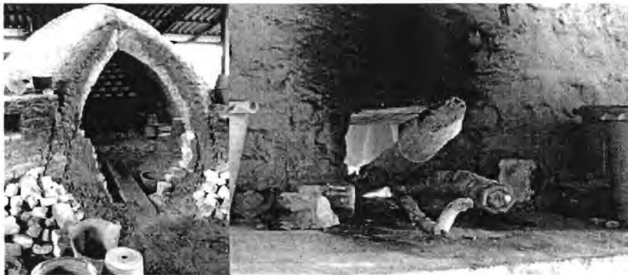
รูปที่ 3.96 การเผาด้วยเตาซัง ของโรงงานเครื่องปั้นดินเผา ตำบลหูกวางอำเภอบรรพตพิสัย จังหวัดนครสวรรค์
