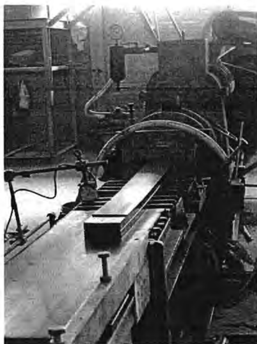
รูปที่ 3.83 การใช้เครื่องรีดดิน ของโรงงานอิฐ ตำบลบางปลาจืด อำเภอป่าโมก จังหวัดอ่างทอง
