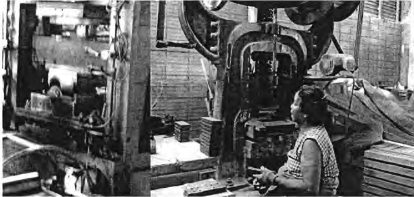
รูปที่ 3.84 การอัดแบบแม่พิมพ์ด้วยเครื่องไฮดรอลิก ของโรงงานอิฐ ตำบลบางปลาгод อำเภอป่าโมก จังหวัดอ่างทอง
