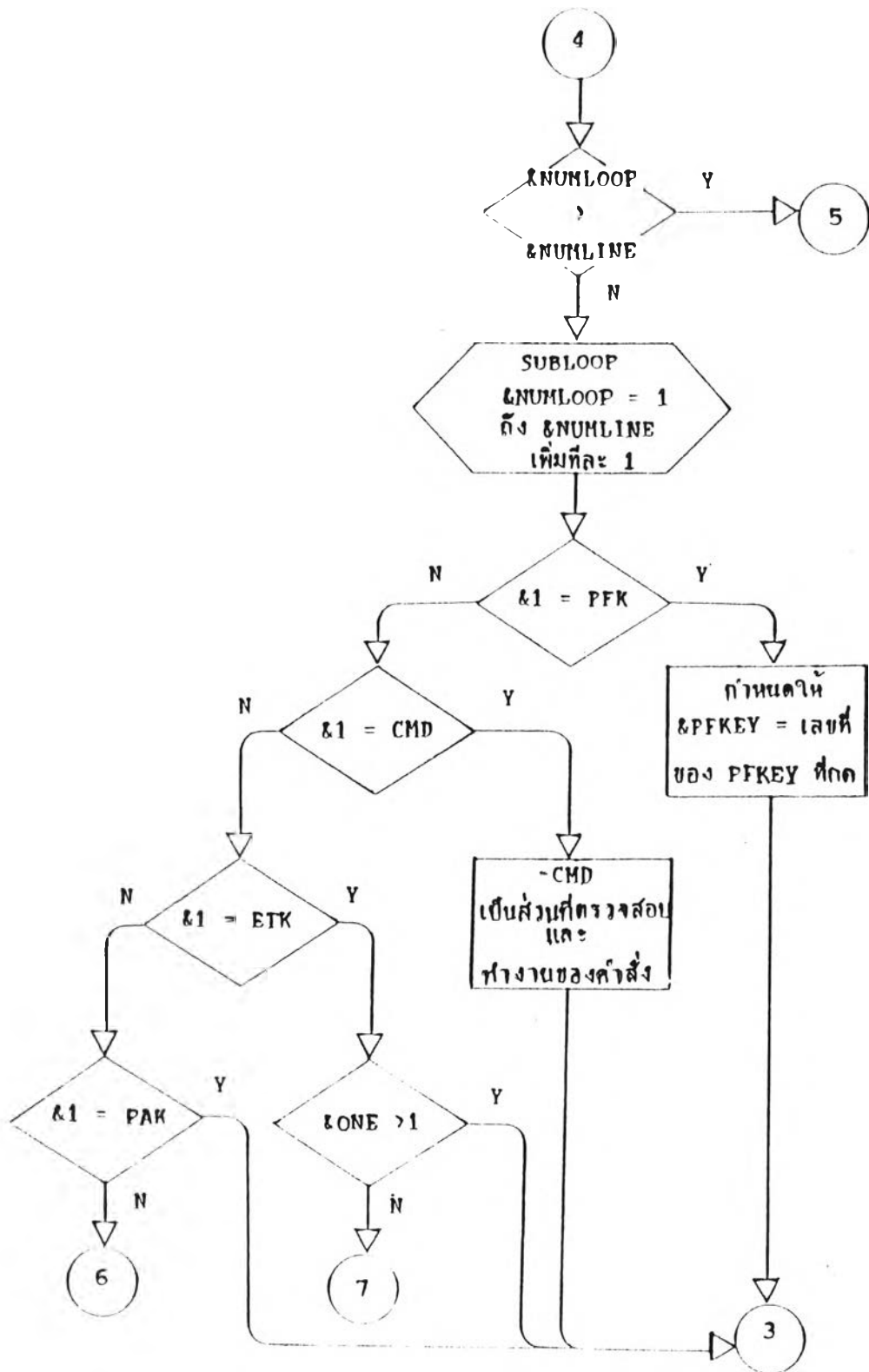
ผังงานที่ 5.3 แสดงการดำเนินงานของ Thaiedit Xedit A (ต่อ)
