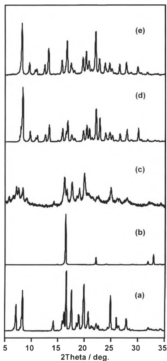
Figure 6. Diffraction patterns of (a) 1 , (b) CuCl 2 , (c) 1 -CuCl 2 , (d) 3 , and (e) 3 -CuCl 2 .
