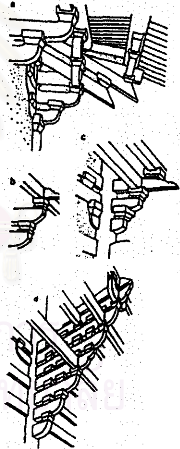
ภาพที่ 6 โครงสร้างเสาและค้ำยัน พร้อมส่วนประกอบต่างๆ ภาพที่ 7 รายละเอียดแสดงถึงกระจับรับชายคาแบบต่างๆ ที่มา : อรุณี ปาณินท์, "การศึกษาเปรียบเทียบวัดจีนในกรุงเทพฯ", (งานวิจัยเสนอต่อคณะสถาปัตยกรรมศาสตร์ มหาวิทยาลัยศิลปากร, 2533), หน้า 133-134
