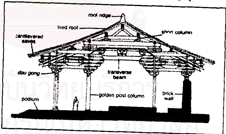
ภาพที่ 4 รูปตัดของวัดทุ่งกุสี แสดงถึงส่วนประกอบที่สำคัญของอาคาร ฐาน ตัวอาคาร และหลังคา รวมทั้งตำแหน่งของแท่นบูชา ที่มา : เอวิสัน , ตำนานวัดและเทพเจ้าจีน , หน้า 40.
