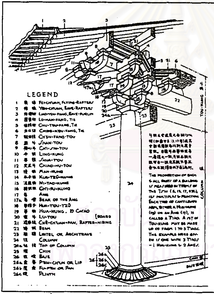
ภาพที่ 6 โครงสร้างเสาและค้ำยัน พร้อมส่วนประกอบต่างๆ ภาพที่ 7 รายละเอียดแสดงถึงกระจับรับชายคาแบบต่างๆ ที่มา : อรุณี ปาณินท์, "การศึกษาเปรียบเทียบวัดจีนในกรุงเทพฯ", (งานวิจัยเสนอต่อคณะสถาปัตยกรรมศาสตร์ มหาวิทยาลัยศิลปากร, 2533), หน้า 133-134
