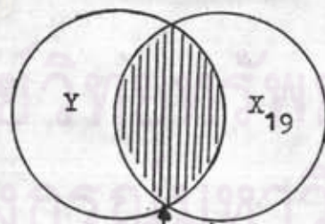
ความแปรปรวนใน Y ซึ่งอธิบายได้ด้วย X_{19}
