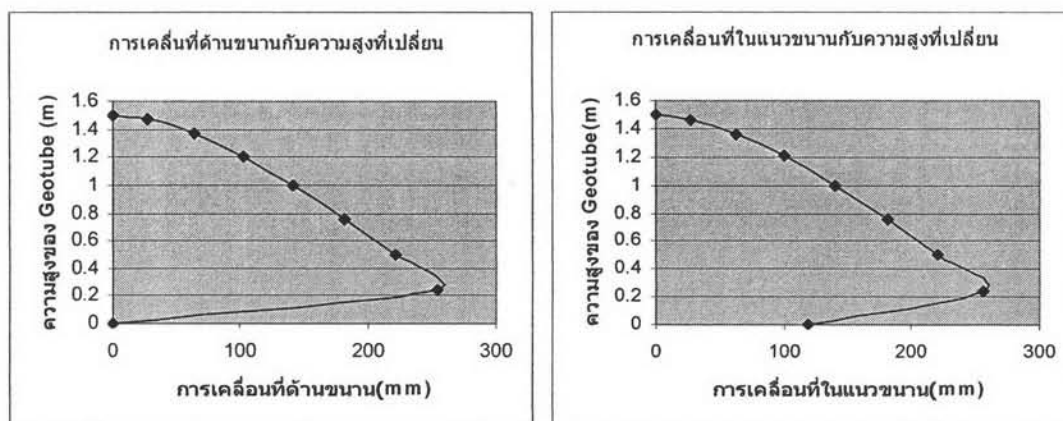
รูปที่ 5.1 (ก) ค่า EA มีค่า 500 kN/m (ข) ค่า E มีค่า 10000 kN/m
