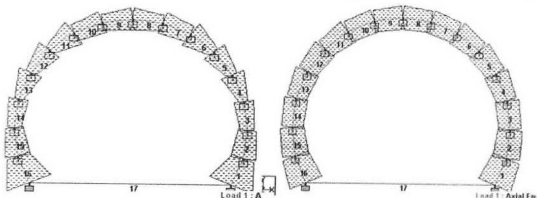
รูปที่ 5.2 (ก)ค่า EA มีค่า 500 kN/m (ข)ค่า E มีค่า 10000 kN/m
