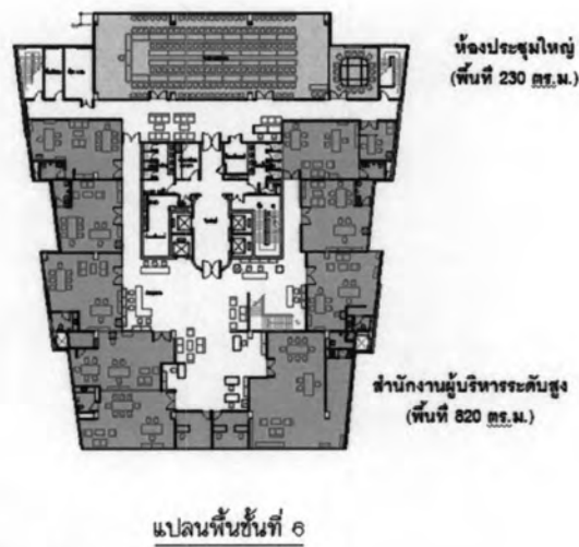
รูปภาพที่ 3.7 แปลนพื้นที่ 6 อาคารสำนักงานใหญ่
