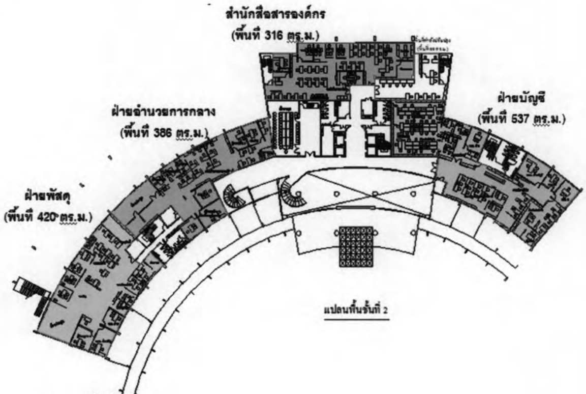
รูปภาพที่ 3.3 ผังพื้นที่ชั้นที่ 2 อาคารสำนักงานใหญ่
