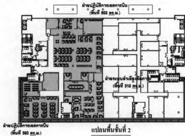
รูปภาพที่ 3.41 ผังพื้นที่ 2 อาคารสำนักงานปฏิบัติการท่าอากาศยานสุวรรณภูมิ
