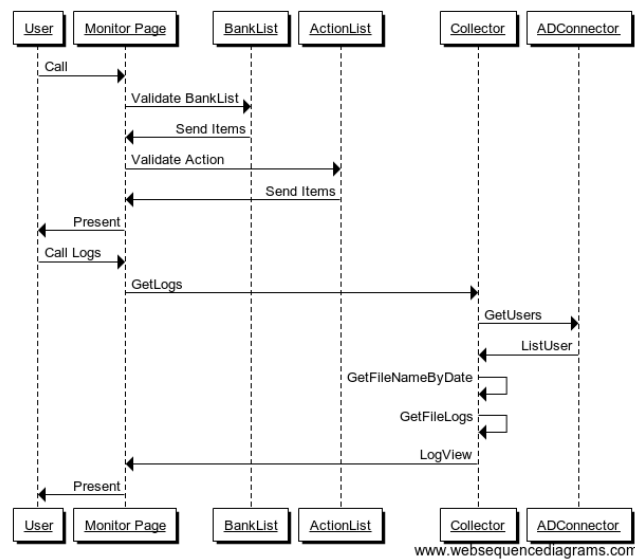
รูปที่ 9 Sequence Diagram ฟังก์ชันหน้า Monitor ที่ได้จากการผลิต
