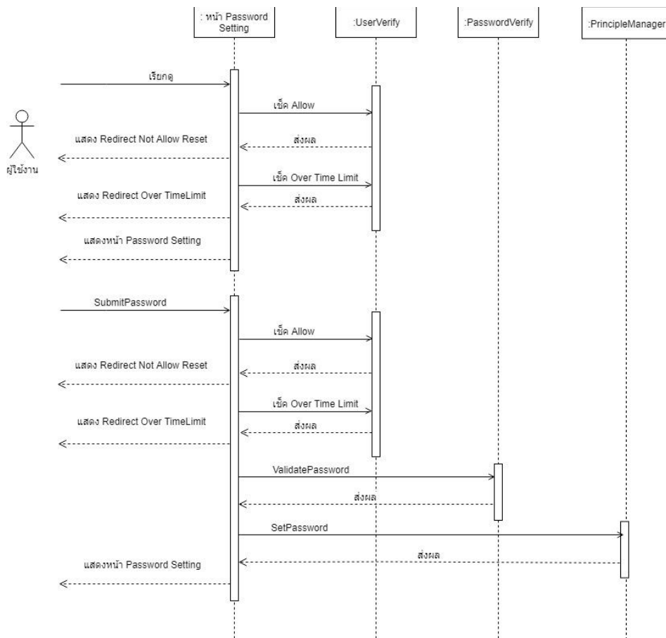
รูปที่ 14 Sequence Diagram ฟังก์ชันหน้า Password Management จากเอกสาร FS จุฬาลงกรณ์มหาวิทยาลัย CHULALONGKORN UNIVERSITY
