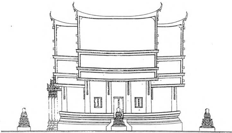
(ภาพถ่ายเส้นแสดงตัวเรือนพระอุโบสถวัดสระบัวมาตราส่วน 1:200)
