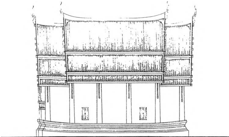
(ภาพถ่ายเส้นแสดงตัวเรือนพระอุโบสถวัดสระบัวมาตราส่วน 1:200)
