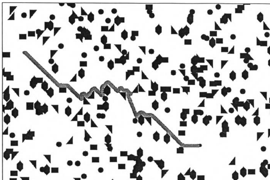
รูปที่ ข.10 แสดงการเคลื่อนที่ของหุ่นยนต์ซึ่งควบคุมโดยคำตอบที่ได้จากการทดลองที่ 5
