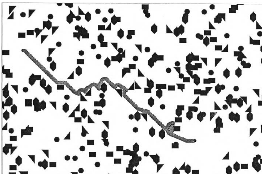
รูปที่ ข.18 แสดงการเคลื่อนที่ของหุ่นยนต์ซึ่งควบคุมโดยคำตอบที่ได้จากการทดลองที่ 9
