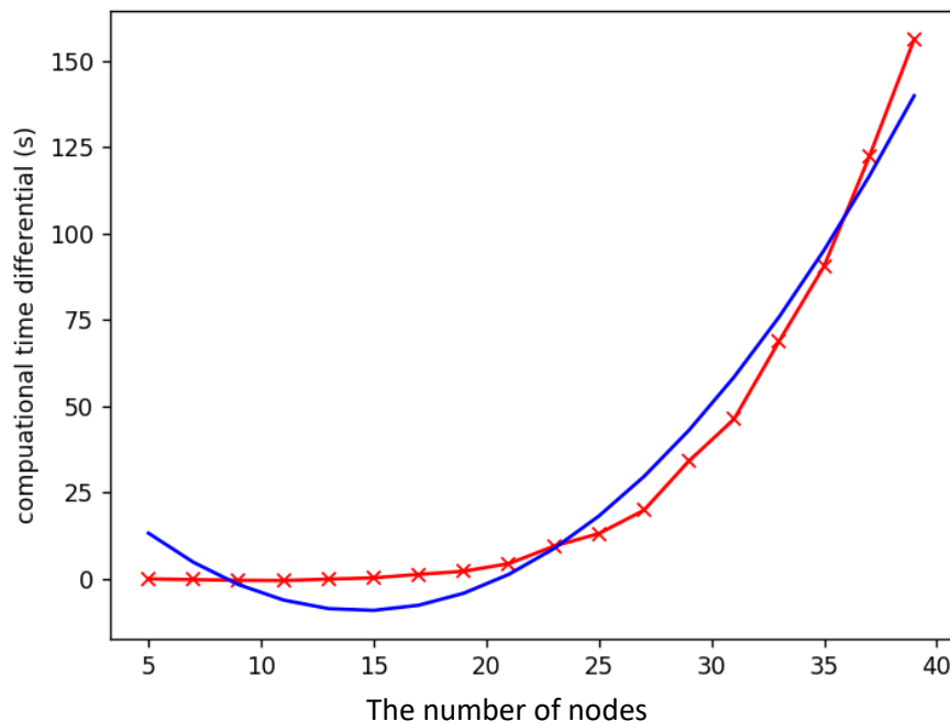
รูปที่ 28 กราฟผลต่างด้านเวลาในการหาคำตอบของขั้นตอนวิธีเชิงพันธุกรรม และการถดถอยแบบพหุนาม
