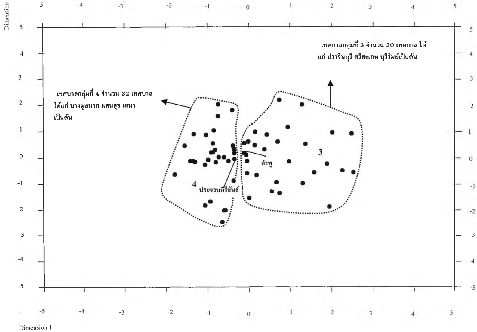
แผนภูมิที่ 5.4 การกระจายตัวของเทศบาลนครและเทศบาลเมือง 62 แห่งบนพื้นระนาบ 2 มิติด้านการแยกย่อยทางสังคม
