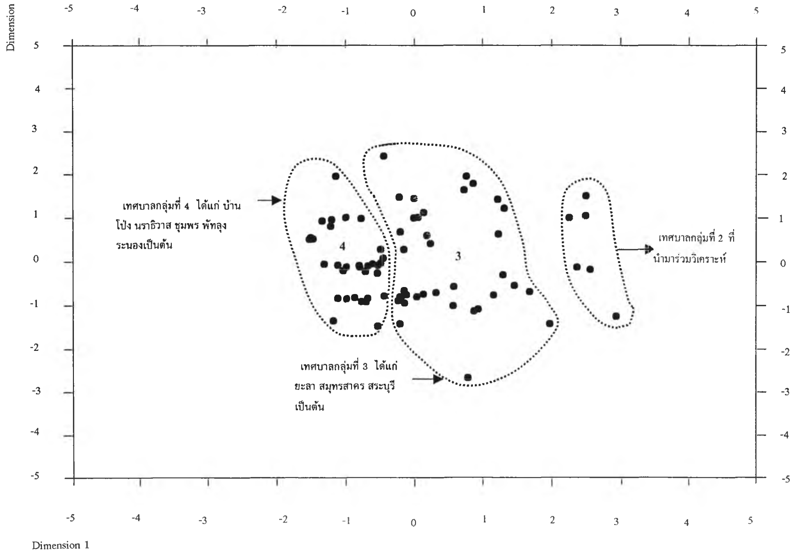
แผนภูมิที่ 5.2 การกระจายตัวของเทศบาลนครและเทศบาลเมือง 75 แห่งบนพื้นระนาบ 2 มิติด้านการแยกย่อยทางเศรษฐกิจ
