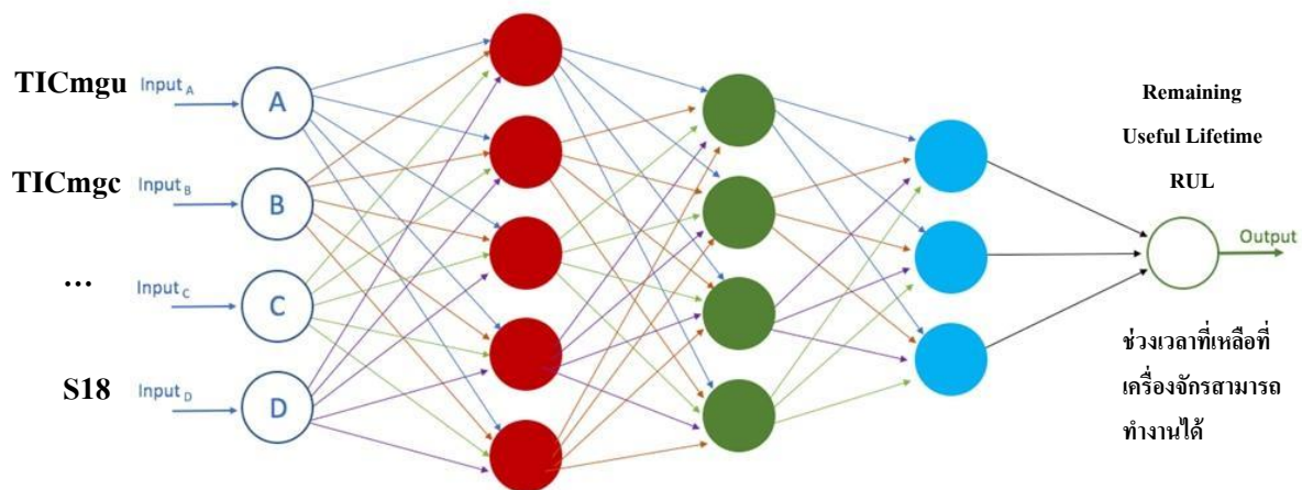
รูปที่ 38 แนวคิดการสร้าง Model Neural network ในงานวิจัยนี้
