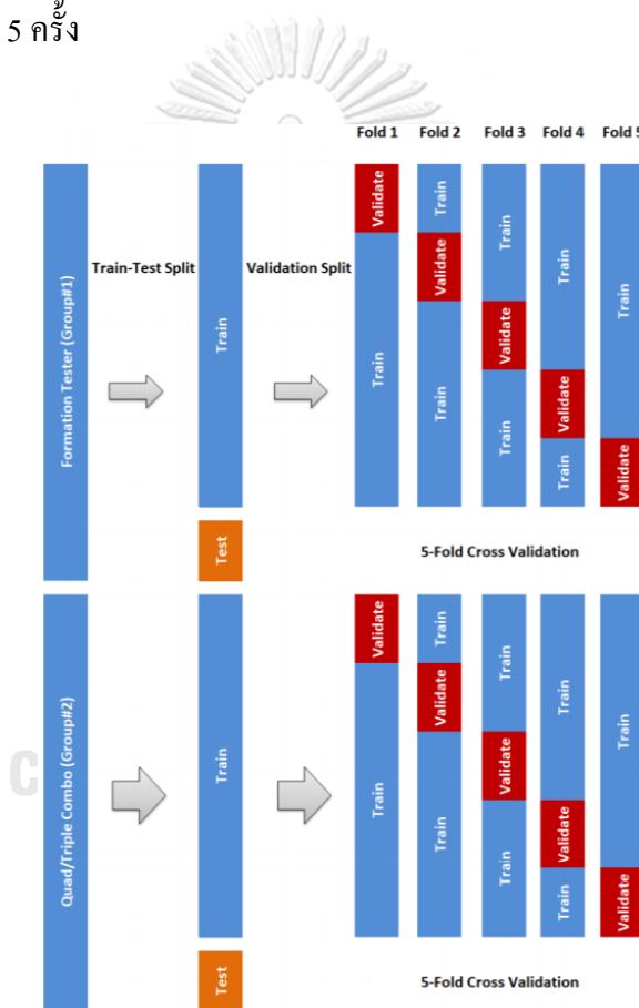
รูปที่ 25 5-Fold Cross validation กับ Training data
