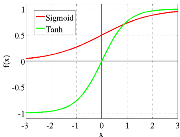
รูปที่ 11 Function การทำงานของ Tanh
