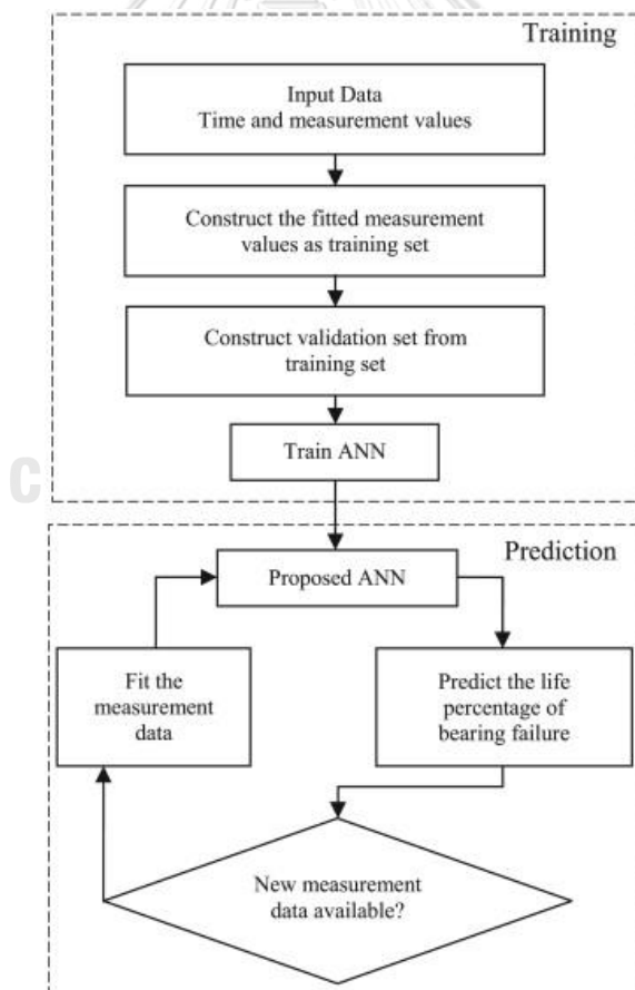
รูปที่ 32 Flow chart การทำ Predictive model
