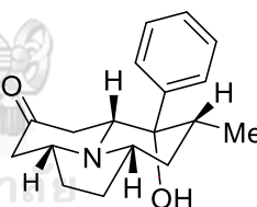
[318] Crepidatumine D
