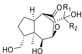
[209] Dendronobilin L, R_1=Me , R_2=CH_2
