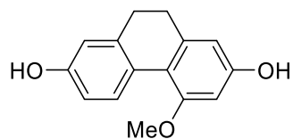
Coelonin [9]
