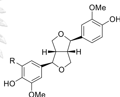
[299] (-)-Medioresinol: R = OMe
