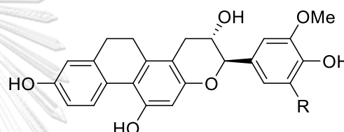
[134] Chrysotoxol A: R = H
