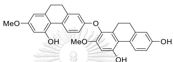
[157] Phoyunnanin E
