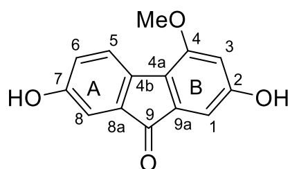
Nobilone [308]
