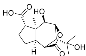
[207] Dendronobilin J
