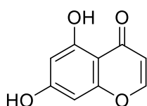
[323] 5,7-Dihydroxy-chromen-4-one
