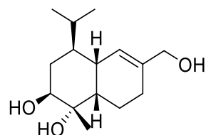
[204] Dendronobilin G
