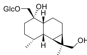
[216] Dendroside E
