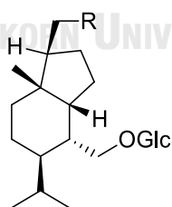
[193] Dendronobiloside A: R = \text{OGlc}
