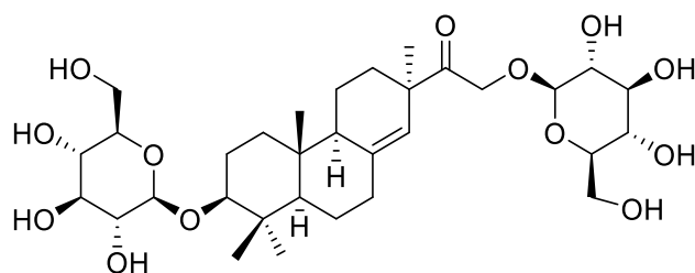
Flifimdioside A [16]
