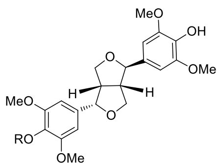
[295] Episingaresinol: R = H
