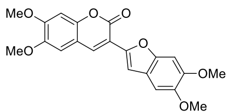
[286] Denthyrsin
