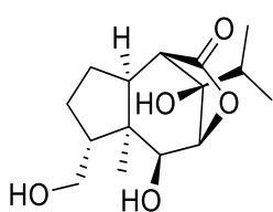
[199] Dendronobilin B
