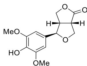
[289] Dendrolactone
