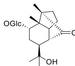
[192] Dendromonilide A
