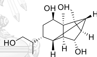
[211] Dendronobilin N
