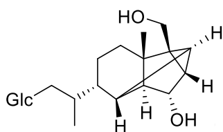
[197] Dendronobiloside E
