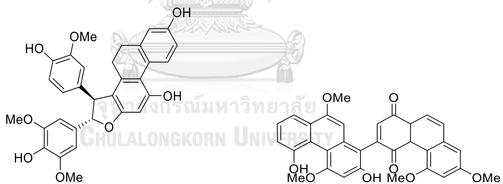
[164] Loddigesiinol J
