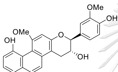
[133] Loddigesiinol B
