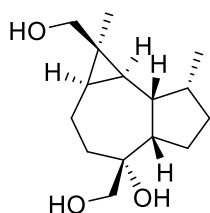
[205] Dendronobilin H
