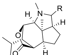
[313] (-)-(1 R ,2 S ,3 R ,4 S ,5 R ,6 S ,9 S ,11 R )-11-carboxymethyldendrobine: R = CH 2 COOH
