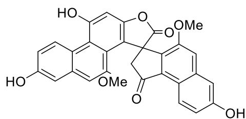
[138] Dendrochrysanene
