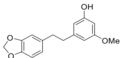
[68] Densiflorol A
