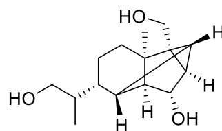
[206] Dendronobilin I
