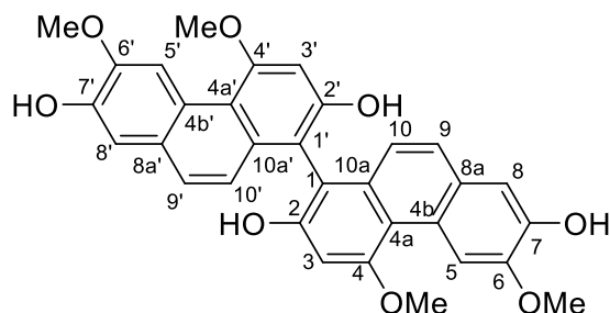
agrostonin [341]
