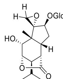
[192] Dendromonilide C
