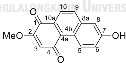
densiflorol B [ 126 ]
