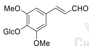
[282] Syringin
