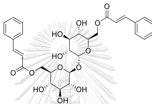
[271] Dendroside
