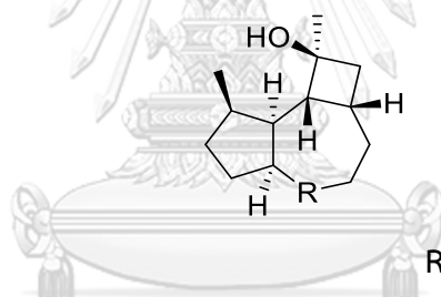
[219] Dendrowardol A
