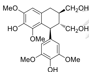
[298] Lyoniresinol
