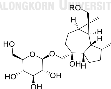
[212] Dendroside A: R = H
