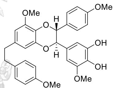
[142] Dendrocandine I
