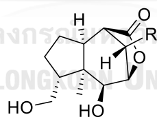
[201] Dendronobilin D; R =
