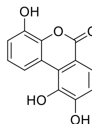
[285] Dendrocoumarin
