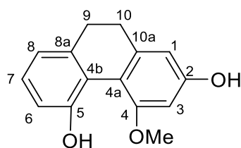
hircinol [94]
