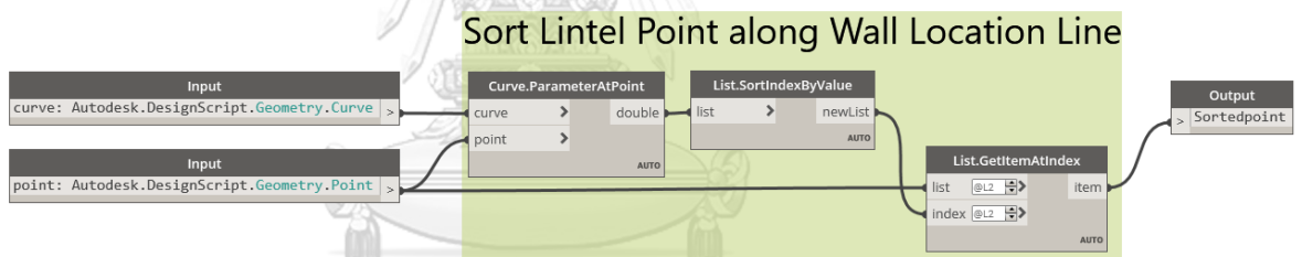
รูปที่ 4.17 กลุ่ม SortLintelPointByWallLocationVector
