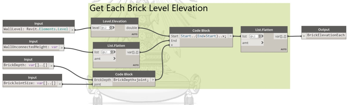
รูปที่ 4.32 กลุ่ม BrickLevelElevationOdd
