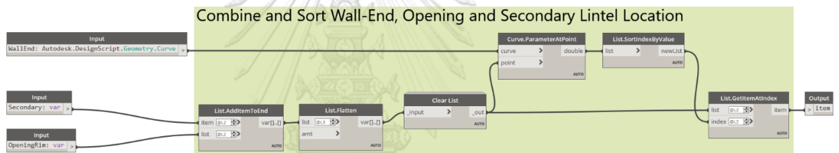
รูปที่ 4.22 กลุ่ม CombineOfWallEnd-OpeningRim-SecondaryPoint
